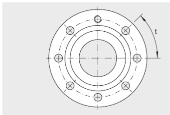
孔的布置
