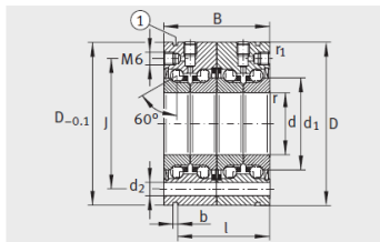
ZKLF.-2RS-2AP
