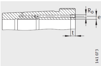
液压拆卸套（后缀 H） 安装尺寸
