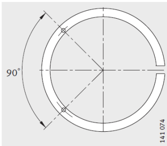
液压拆卸套上用于连接 液压泵的接口
