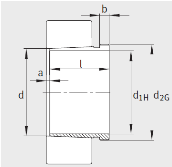
AH240、AH241 锥度为 1：30
