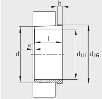
锥度为 1：12
